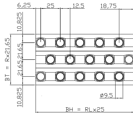
Geometrie 25 x 22; Rohrdurchmesser 9,5 mm
