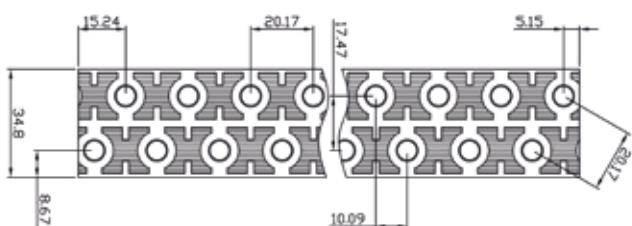
Geometrie 20 x 17; Rohrdurchmesser 6 mm
